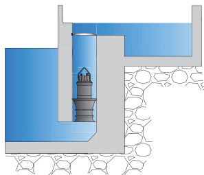
混凝土井筒敞开式： 直接排入渠道，无需拍门。
