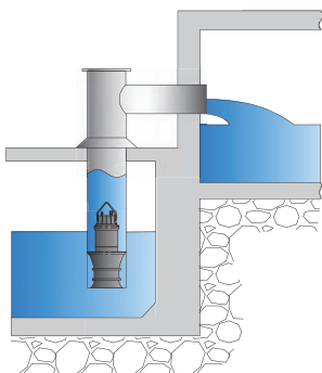
钢制井筒密闭式： 自由出水无需安装拍门。
