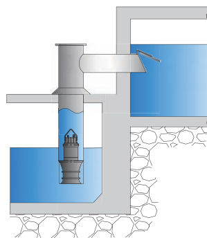
钢制井筒密闭式： 淹没出水需要安装拍门。
