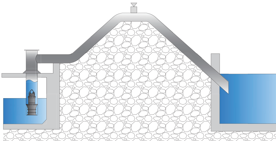
虹吸出水或压力出水
