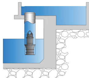
钢制井筒敞开式： 直接排入渠道，无需拍门。
