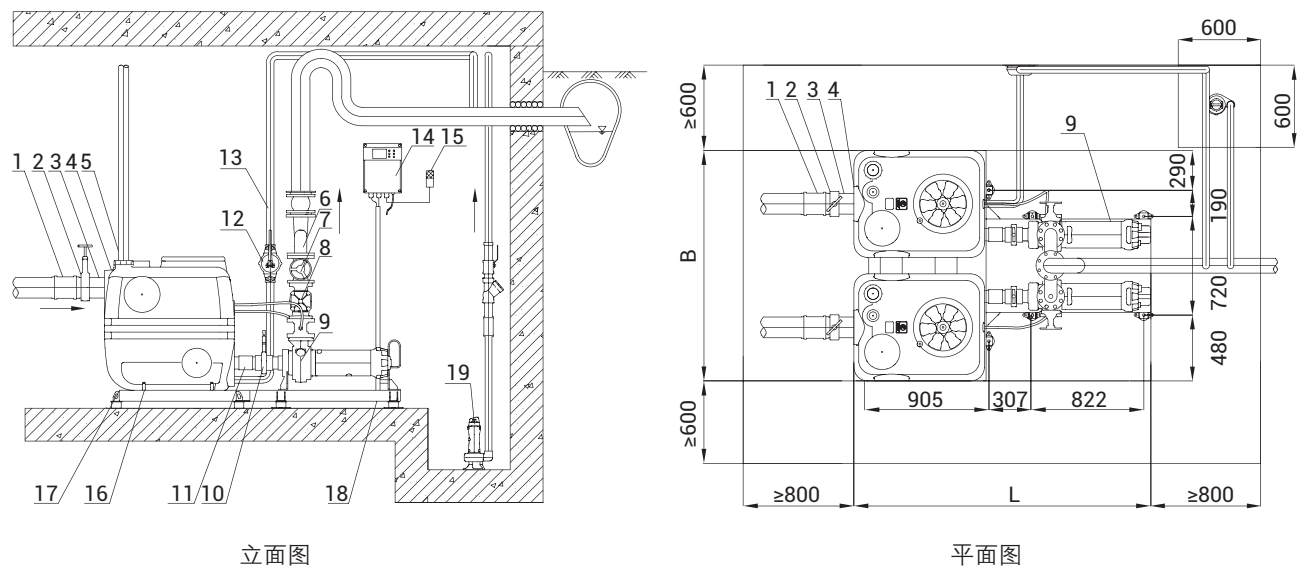
BlueBox 500E 外置式污水提升装置产品安装配置表
