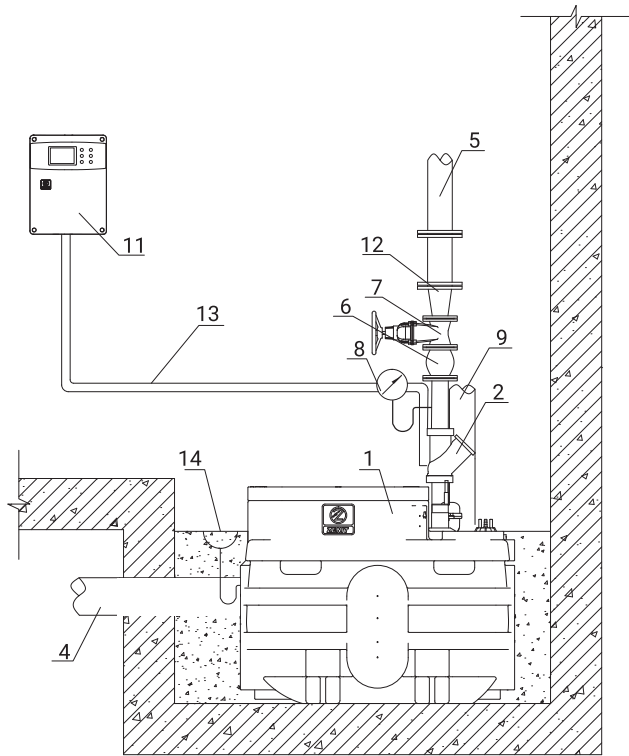
坑内埋置式安装
