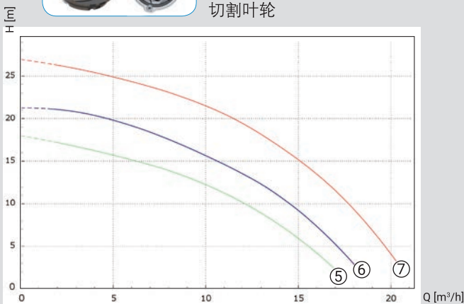
切割叶轮
