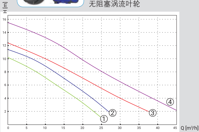
无阻塞涡流叶轮
