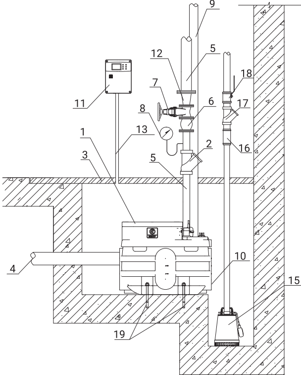
坑内固定式安装
