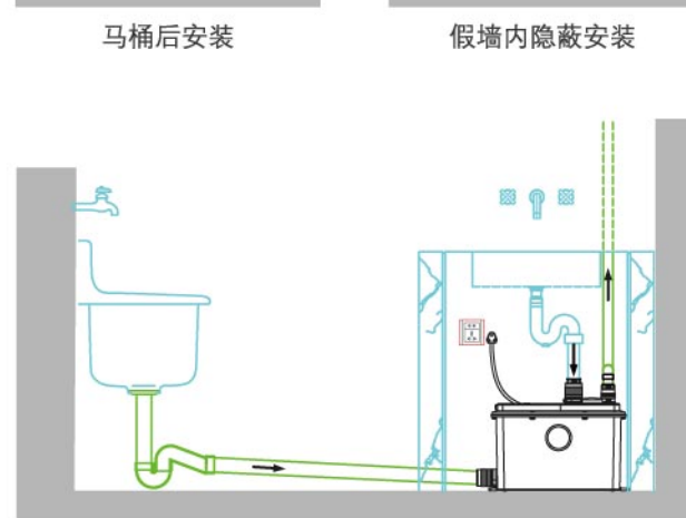
侧面进水安装
